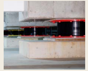
免震ゴム
