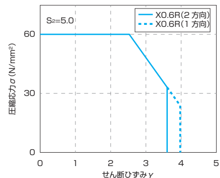
図3：圧縮限界強度の比較例
