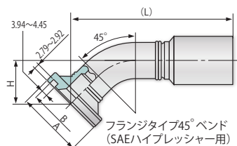
フランジタイプ45° ベンド (SAE/ハイプレッシャー用)
