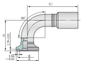
フランジタイプ90° ベンド (SAEスタンダード用)
