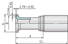
フランジタイプ (SAEハイレッシャー用)
