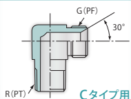
エルボ・アダプタ
